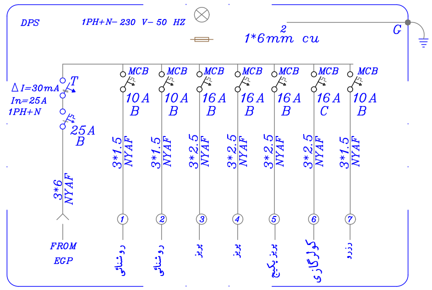
شمای تک خطی تابلو واحد سرایداری
