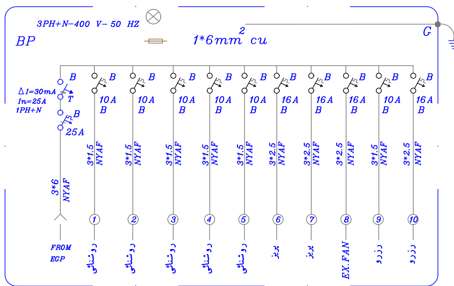
شمای تک خطی تابلو زیرزمین
