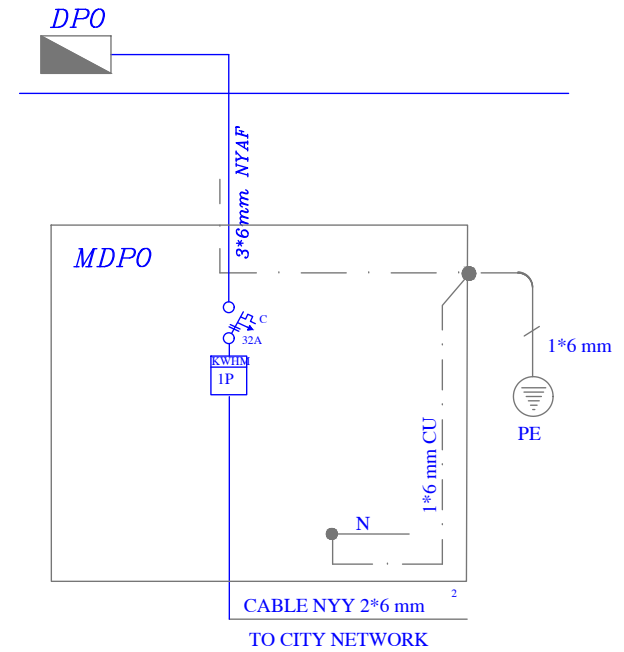
شمای تک خطی تابلو کنتور تجاری
