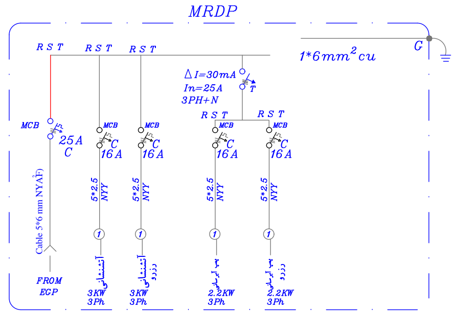
شمای تک خطی تابلو موتورخانه
