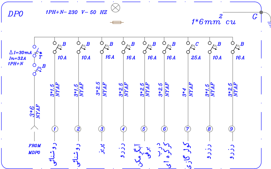
شمای تک خطی تابلو تجاری
