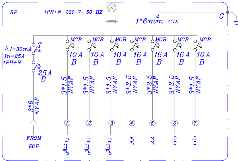
شمای تک خطی تابلو واحد بام
