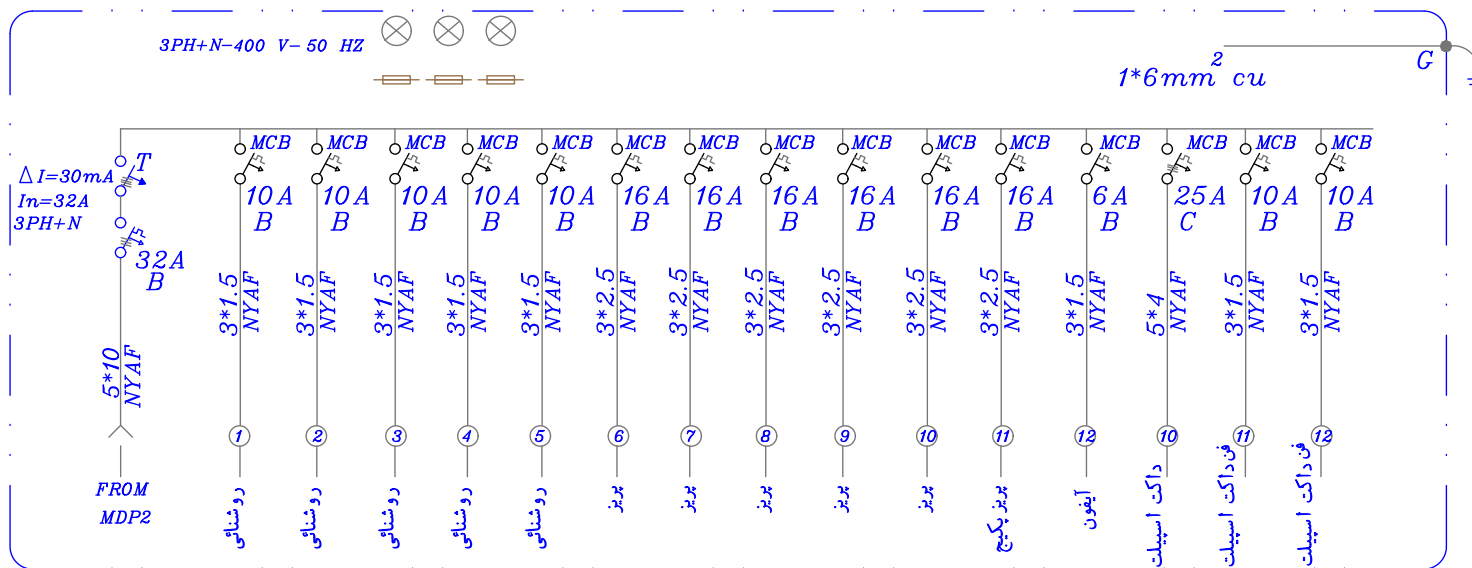
شمای تک خطی تابلو واحد ۲۵ الی ۲۸
