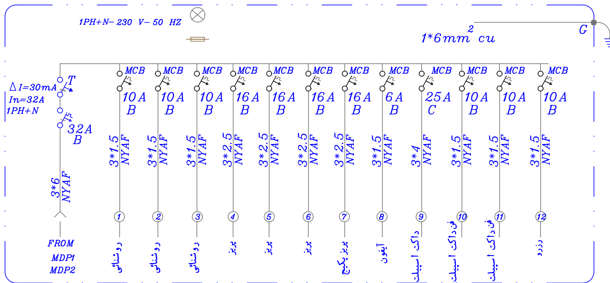
شمای تک خطی تابلو واحد ۱ الی ۲۴
